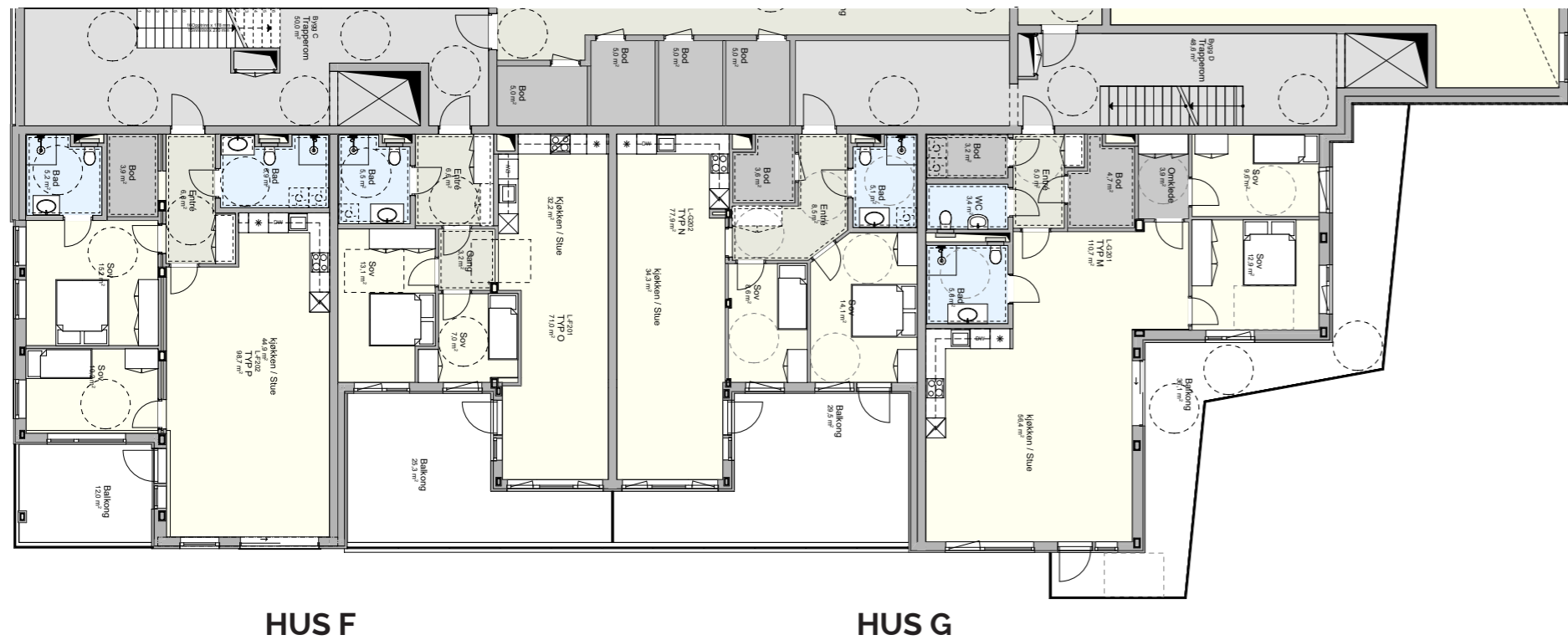
2. etasje
